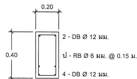
ขยาย B3 SCALE 1:20
