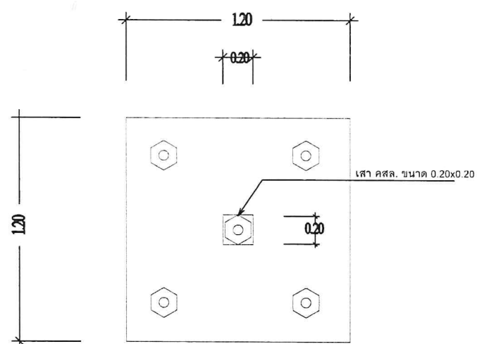
ขยาย S1 SCALE 1:20
