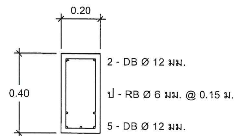
ขยาย B2 SCALE 1:20
