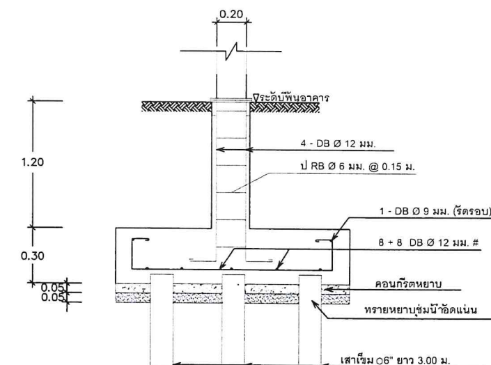
ขยาย F1 SCALE 1:50
