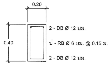
ขยาย B1 SCALE 1:20
