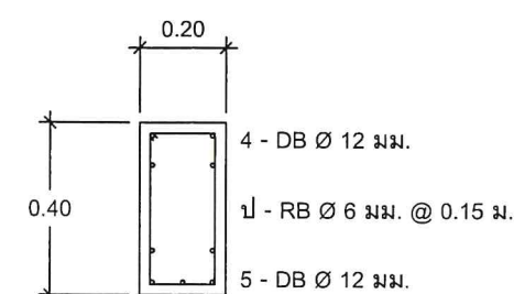
ขยาย B4 SCALE 1:20
