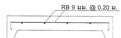
ขยาย GS SCALE 1:20
